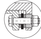
CCR 8) Type
